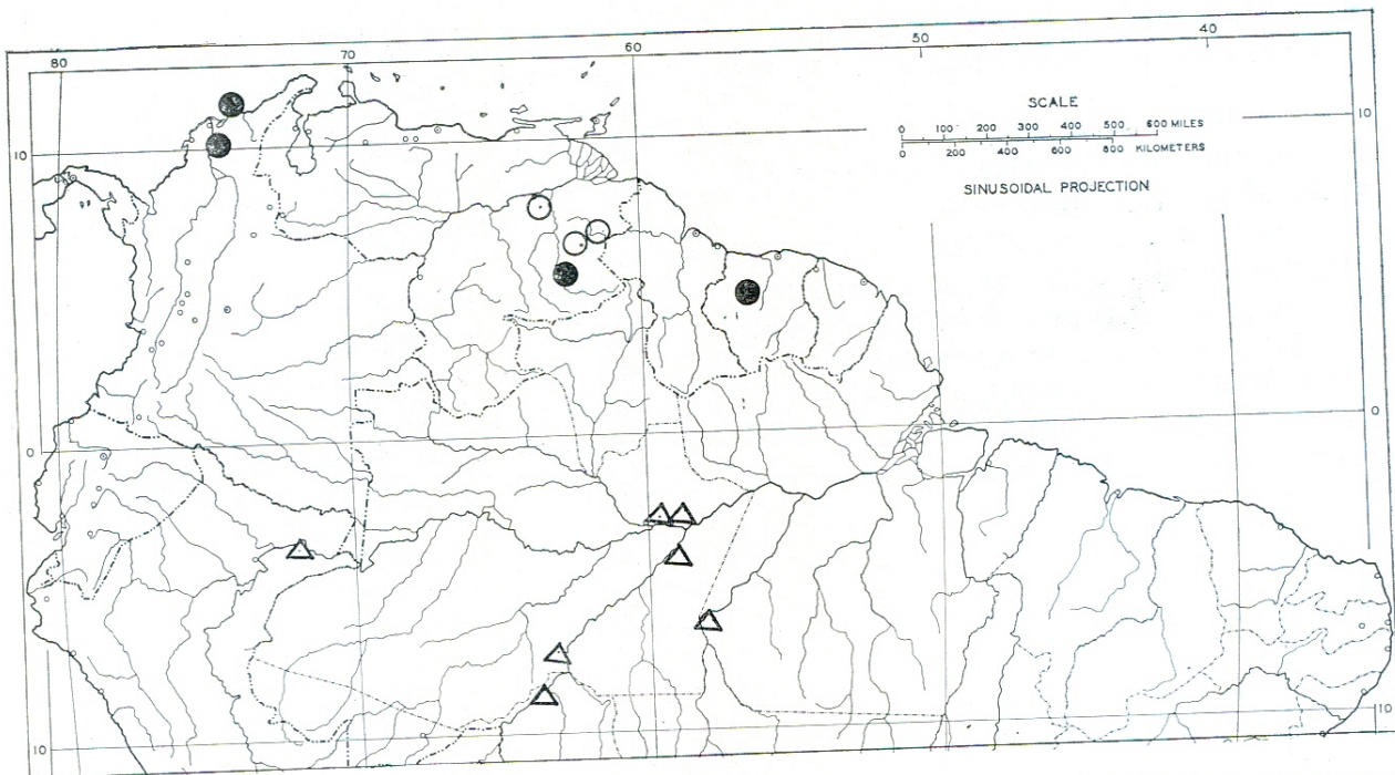
Mapa 4. Distribuição do gênero Sterigmapetalum . ●, S. colombianum ; ○, S. guianense ; △, S. obovatum .
