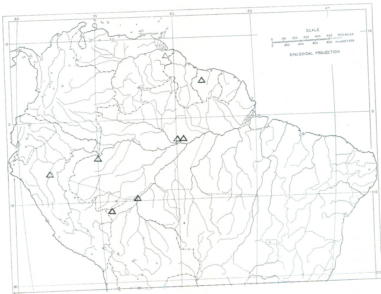
Mapa 2. Distribuição de Cassipourea peruviana .
