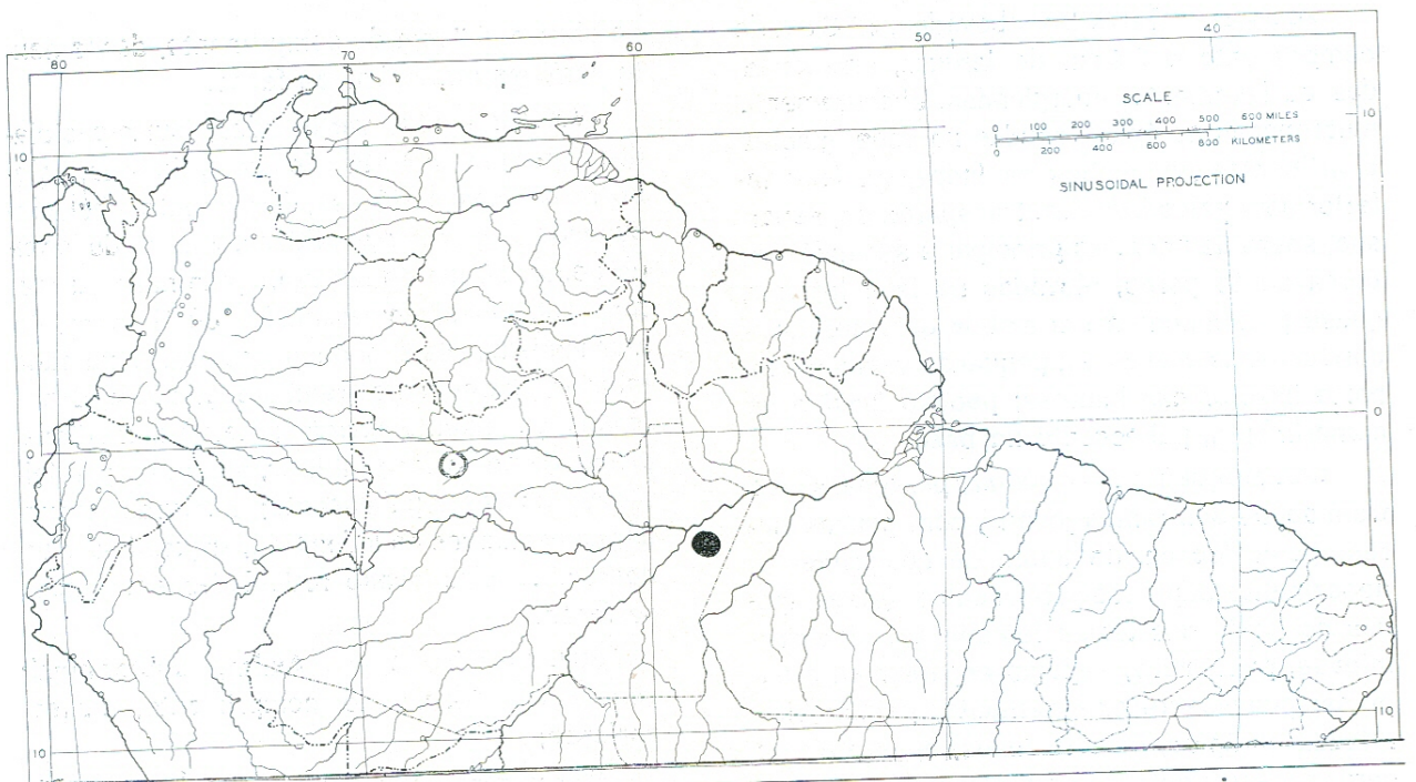
Mapa 5. Distribuição do gênero Polygonanthus . O, P. punctulatus ; ● P. amazonicus .
