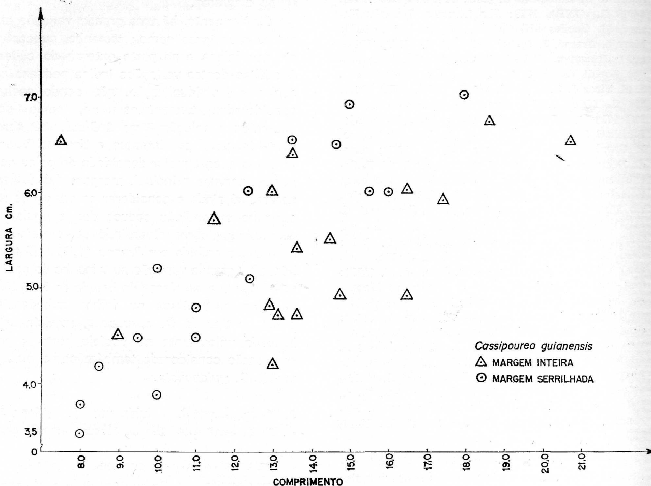
Gráfico. 1. Diagrama pictórico de variação de Cassipourea guianensis Aubl.: — Largura da folha, comprimento da folha e tipo da margem.
