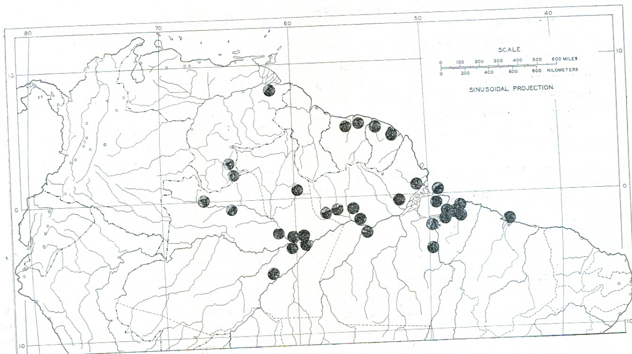
Mapa 3. Distribuição de Cassipourea guianensis .
