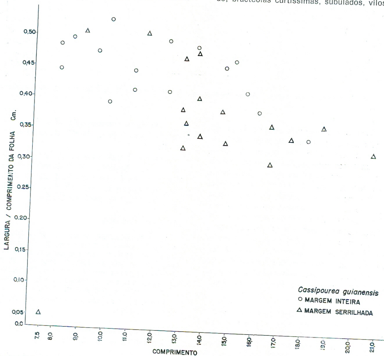
Gráfico. 2. Diagrama pictórico de variação de Cassipourea guianensis Aubl.: — Razão, largura/comprimento de folha, comprimento de folha e tipo de margem. Os diagramas mostram claramente que baseadas nas características analisadas (aquelas usadas pelos autores anteriores para distinguir a nova espécie), Cassipourea serrata não é distinta e nem merece ser reconhecida como variedade taxonômica.
